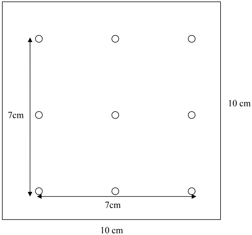
Grundplatte
